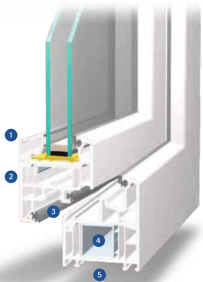
Variante: flächenversetzt
